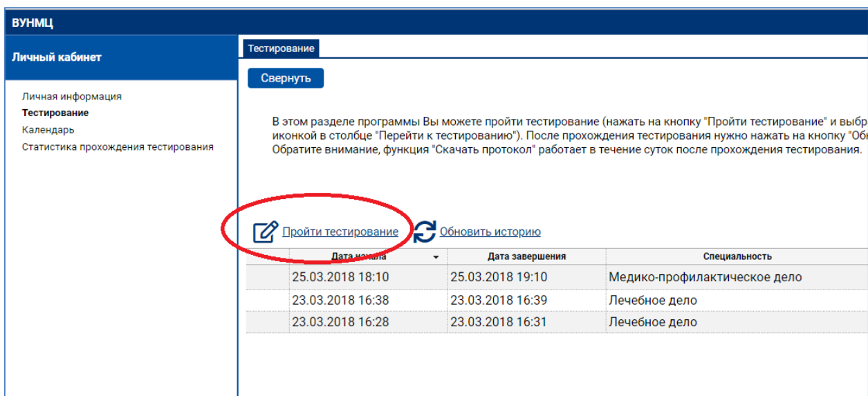
Рис. 11. Страница «Тестирование»
